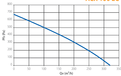
ACX 160 EC
