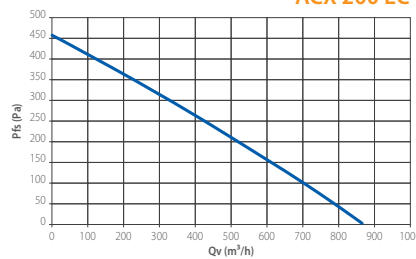
ACX 200 EC
