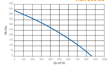
ACX 250 EC
