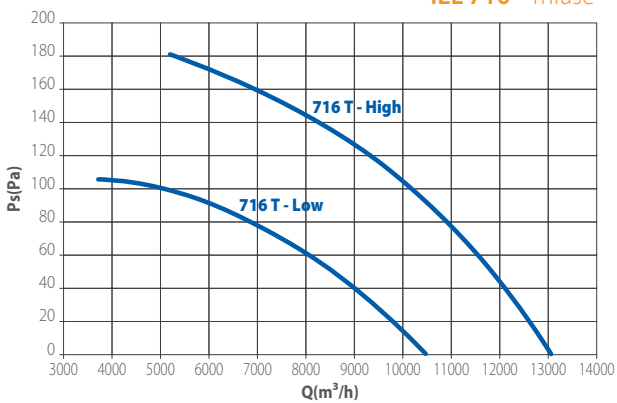
IEL 710 - Trifase
