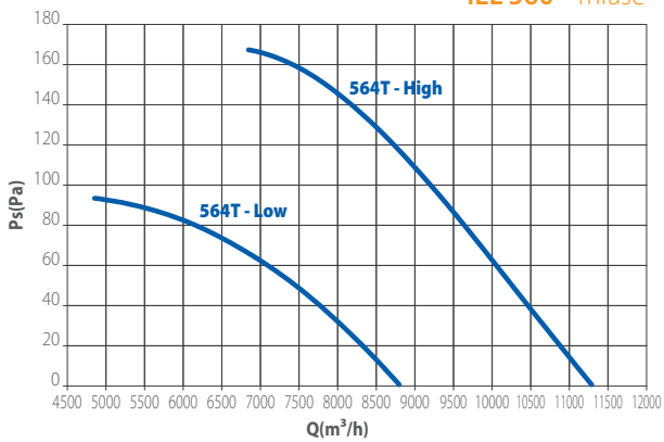
IEL 560 - Trifase
