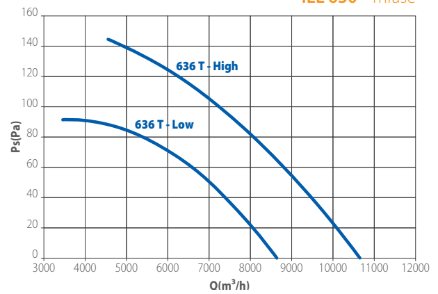
IEL 630 - Trifase
