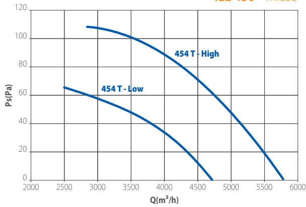
IEL 450 - Trifase
