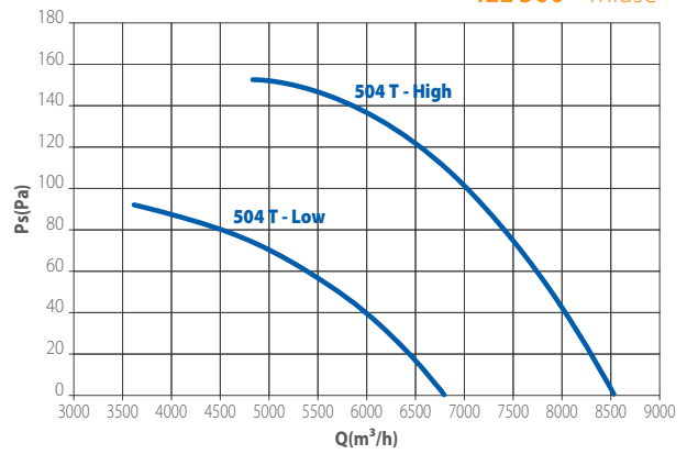
IEL 500 - Trifase
