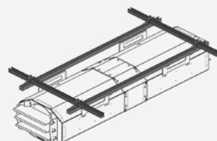
Struttura di fissaggio certificata F400. Adjustable ceiling fixing structure, F400 certified.
