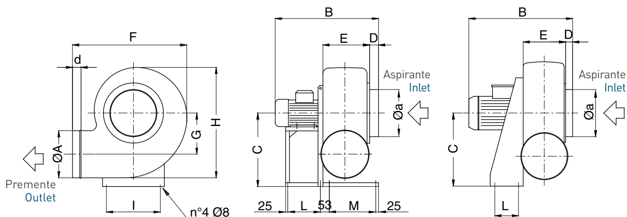
PR AC 50 - 56 - 63
