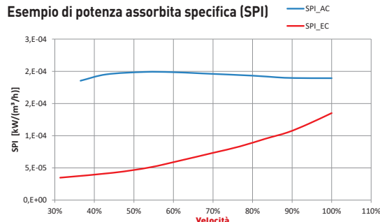
Esempio di potenza assorbita specifica (SPI)
