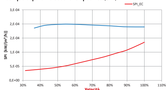
Esempio di potenza assorbita specifica (SPI)
