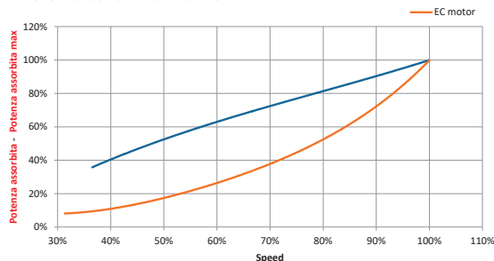
Potenza assorbita relativa
